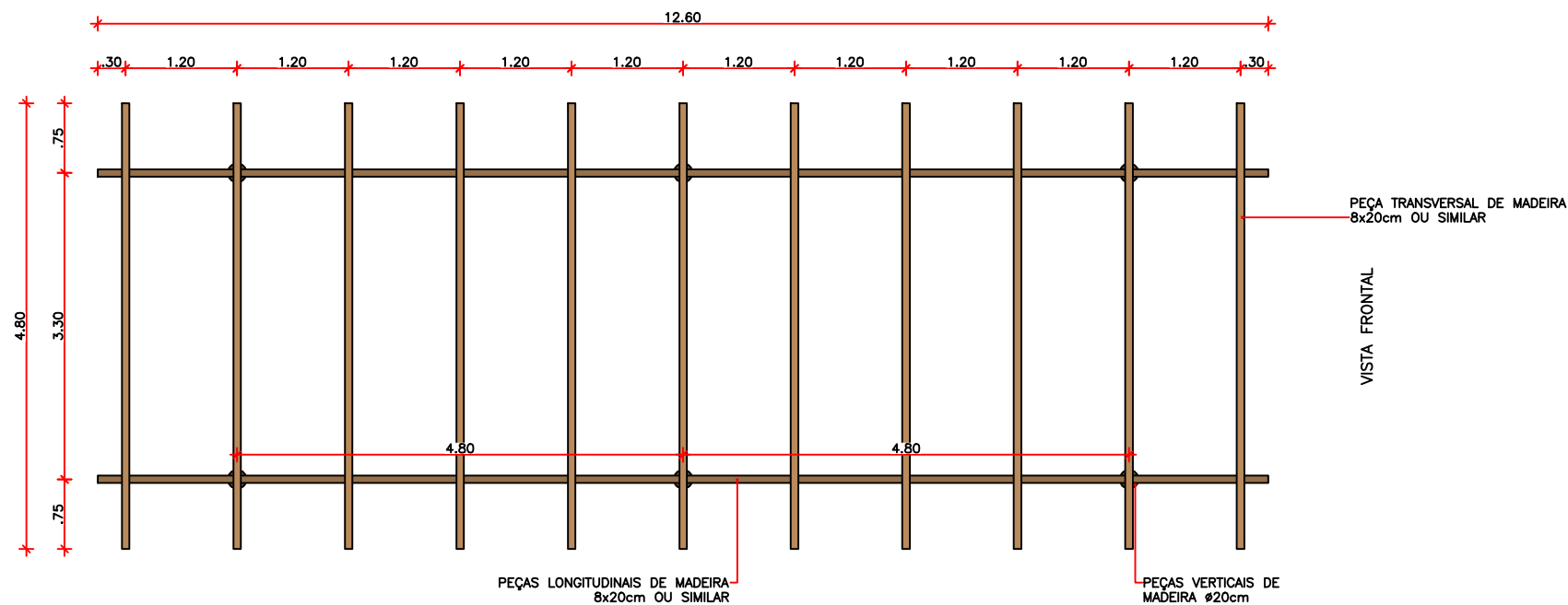
VISTA SUPERIOR ESC.:1/75
