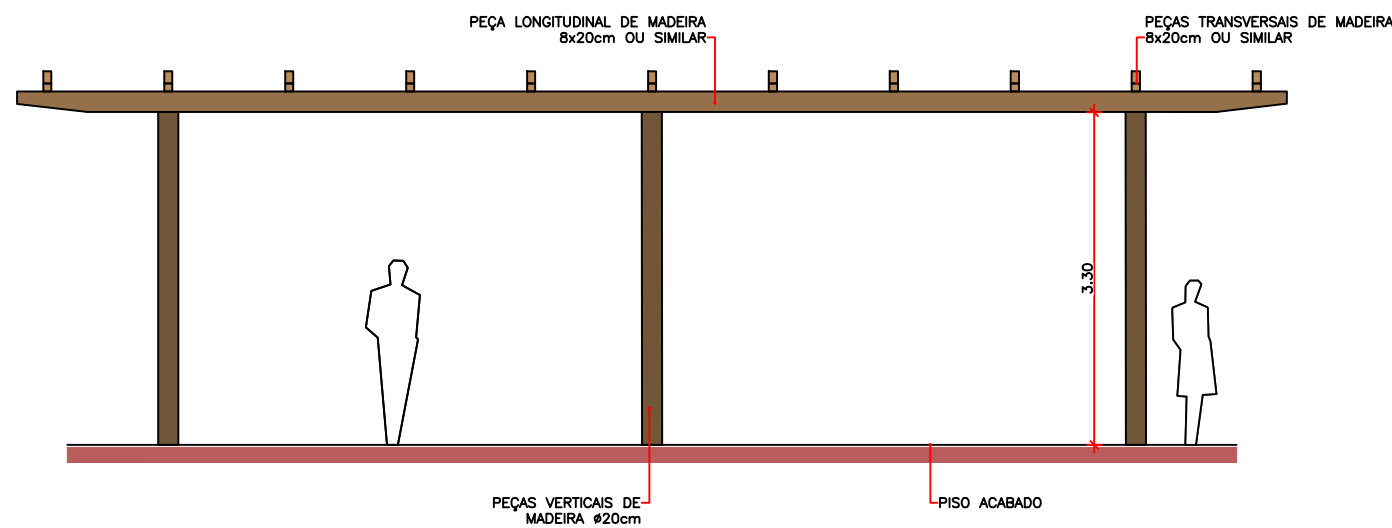
VISTA LATERAL ESC.:1/75
