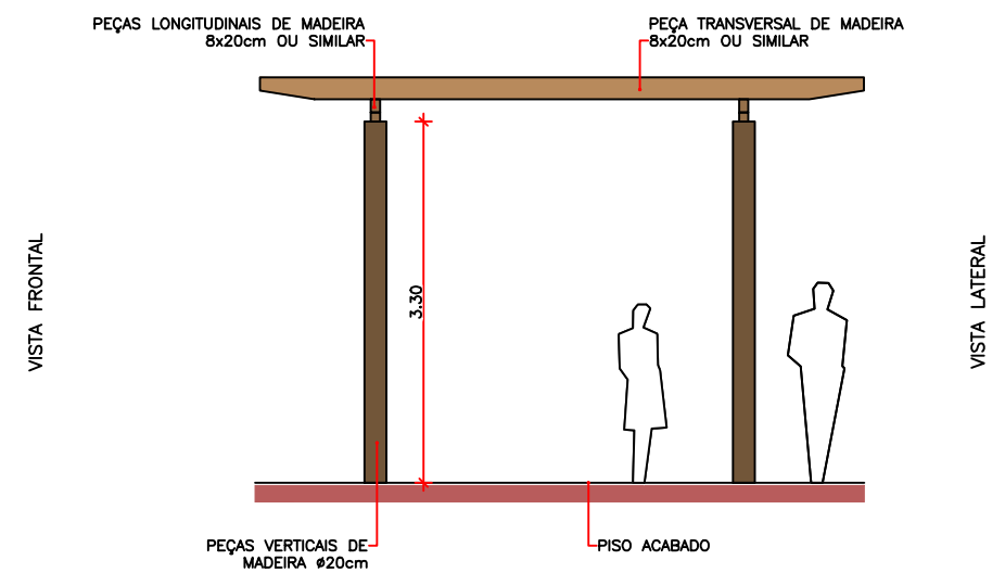
VISTA FRONTAL ESC.:1/75
